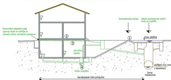
NEPRAVILNO IZVEDEN HIŠNI PRIKLJUČEK NA JAVNO KANALIZACIJO
