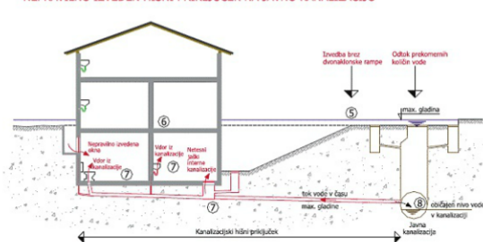
NEPRAVILNO IZVEDEN HIŠNI PRIKLJUČEK NA JAVNO KANALIZACIJO
